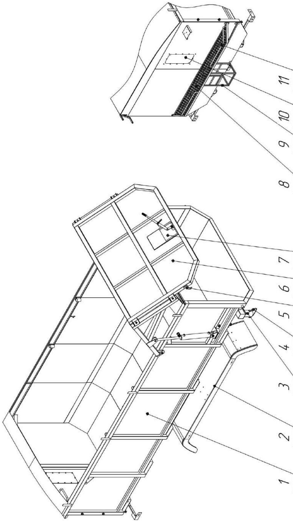
1-кузов; 2-крило; 3-кульова опора кузова; 4-фіксатор; 5-захват; 6-задній борт; 7-шиберна засувка; 8-площадка; 9-драбина; 10-оглядове вікно; 11-поручень
