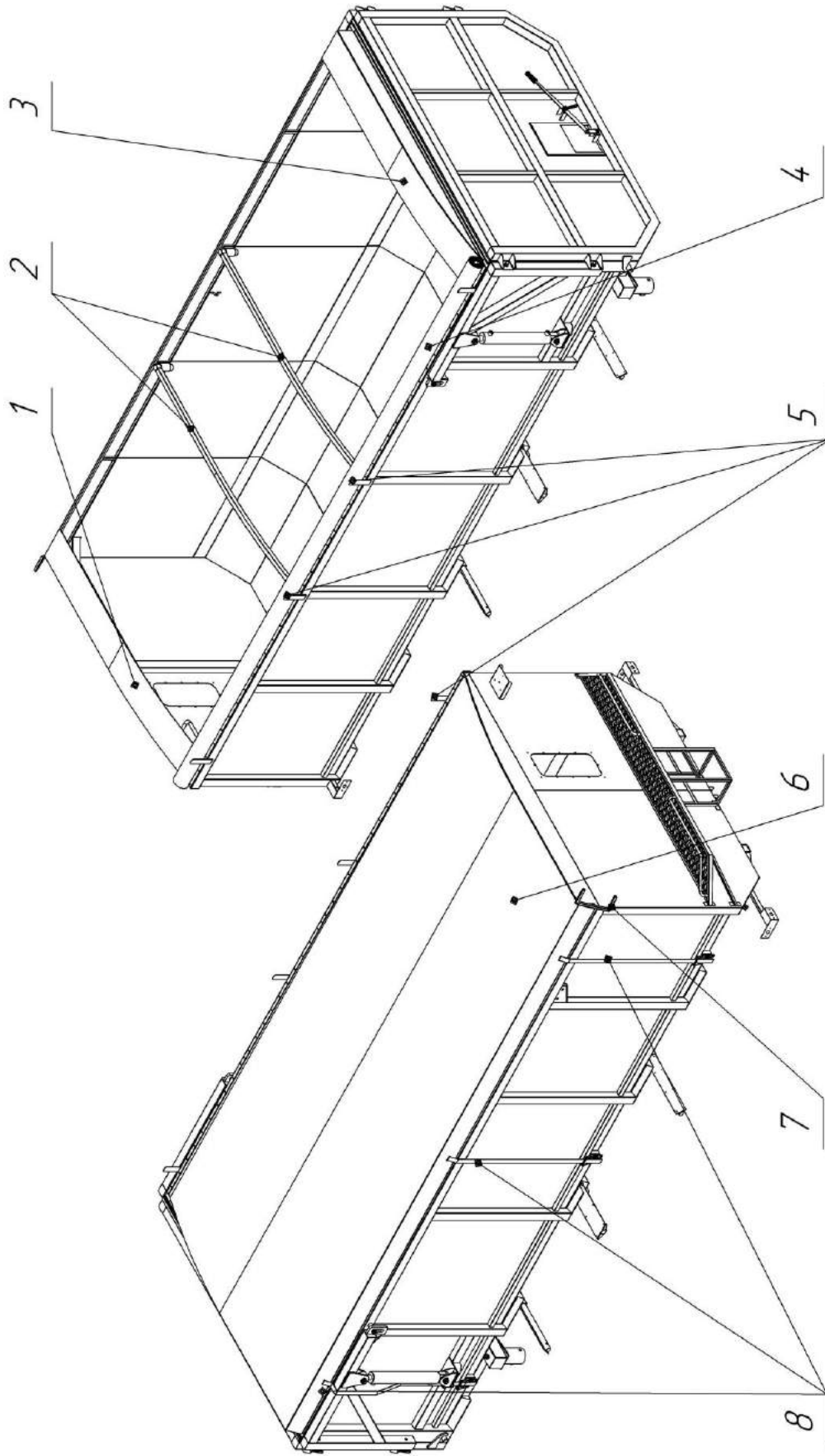
1 -передня напрямлююча; 2-дуги; 3-задня напрямлююча; 4-тент в складеному стані; 5-обмежувач; 6-тент в розкладеному стані; 7-ручка; 8-ремені з натяжними механізмами
